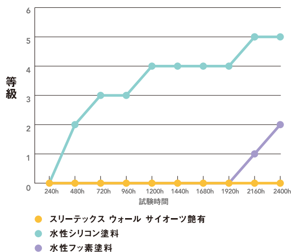
白亜化度 (S-UV)
