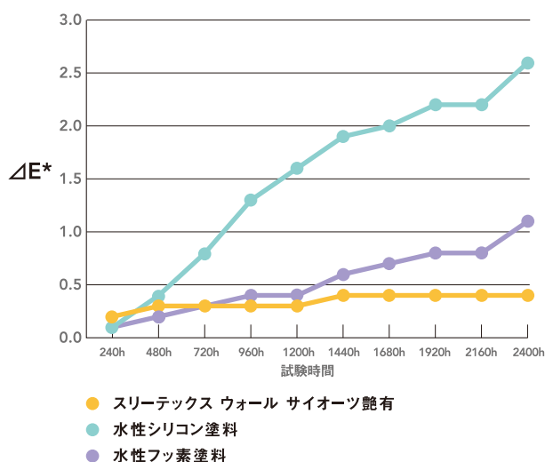
促進耐候性 (S-UV)
